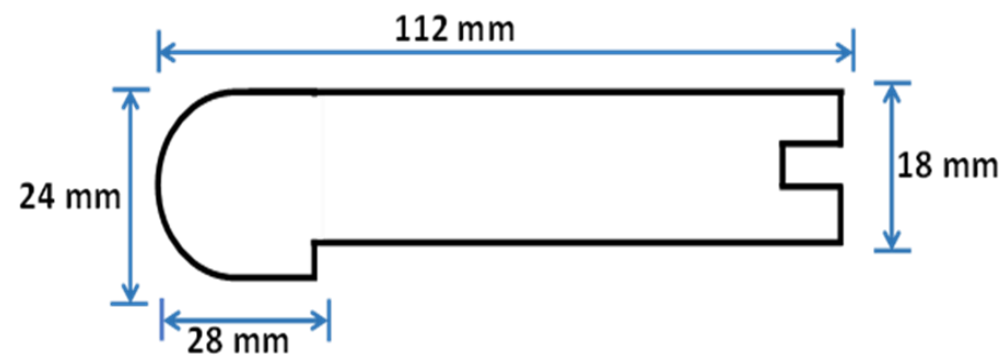
ENG HWD STAIRNOSE(FLUSH)
